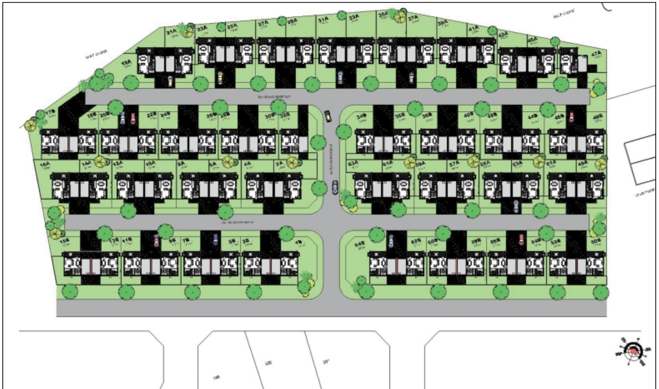
SITE PLAN 1:400 A2
